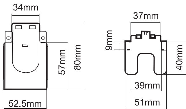
取付金具
